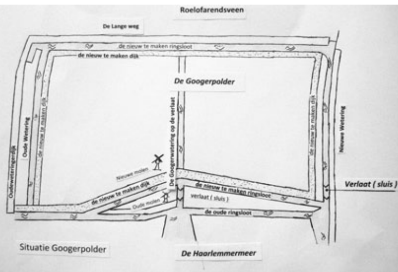
De situatietekening, gemaakt voor het plan van aanpak voor het vervenen van de Googerpolder.
